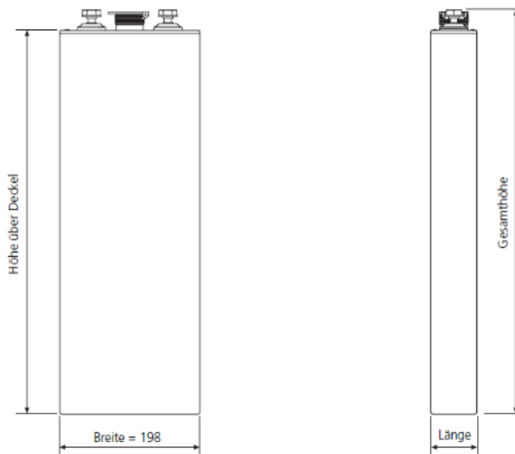
Maßskizze für SPzS-Batteriezelle
